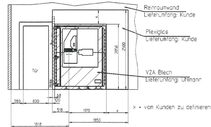
Ansicht von B
